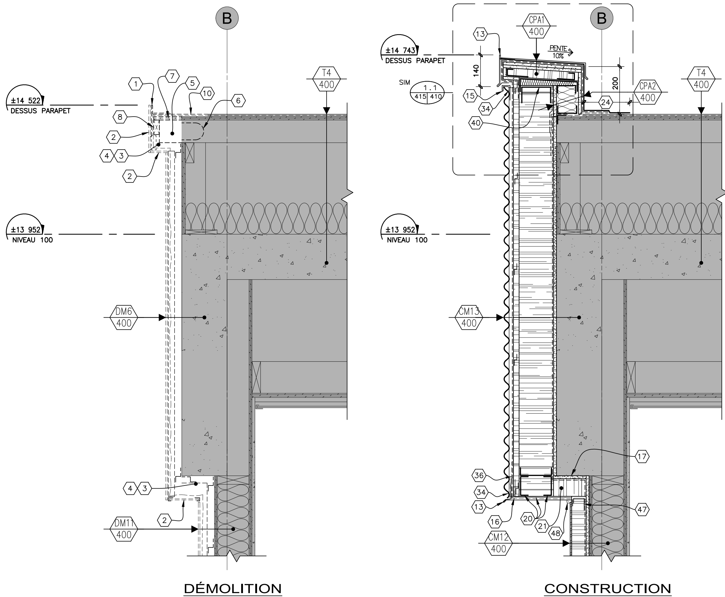
29 DÉTAIL TYPE PARAPET 407 415 1:10mm (GARAGE AMBULANCE)
