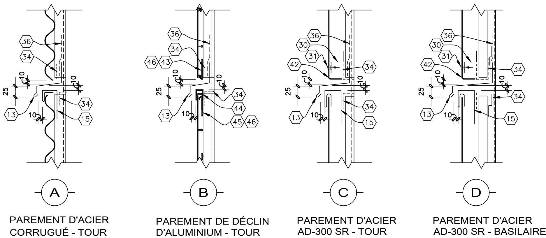
DÉTAILS TYPES DE COMPARTIMENTATION 1:5mm
