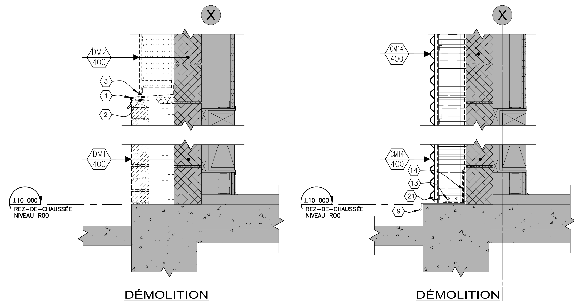
26 DÉTAIL TYPE 406,407 414 1:10mm (ADMINISTRATION)
