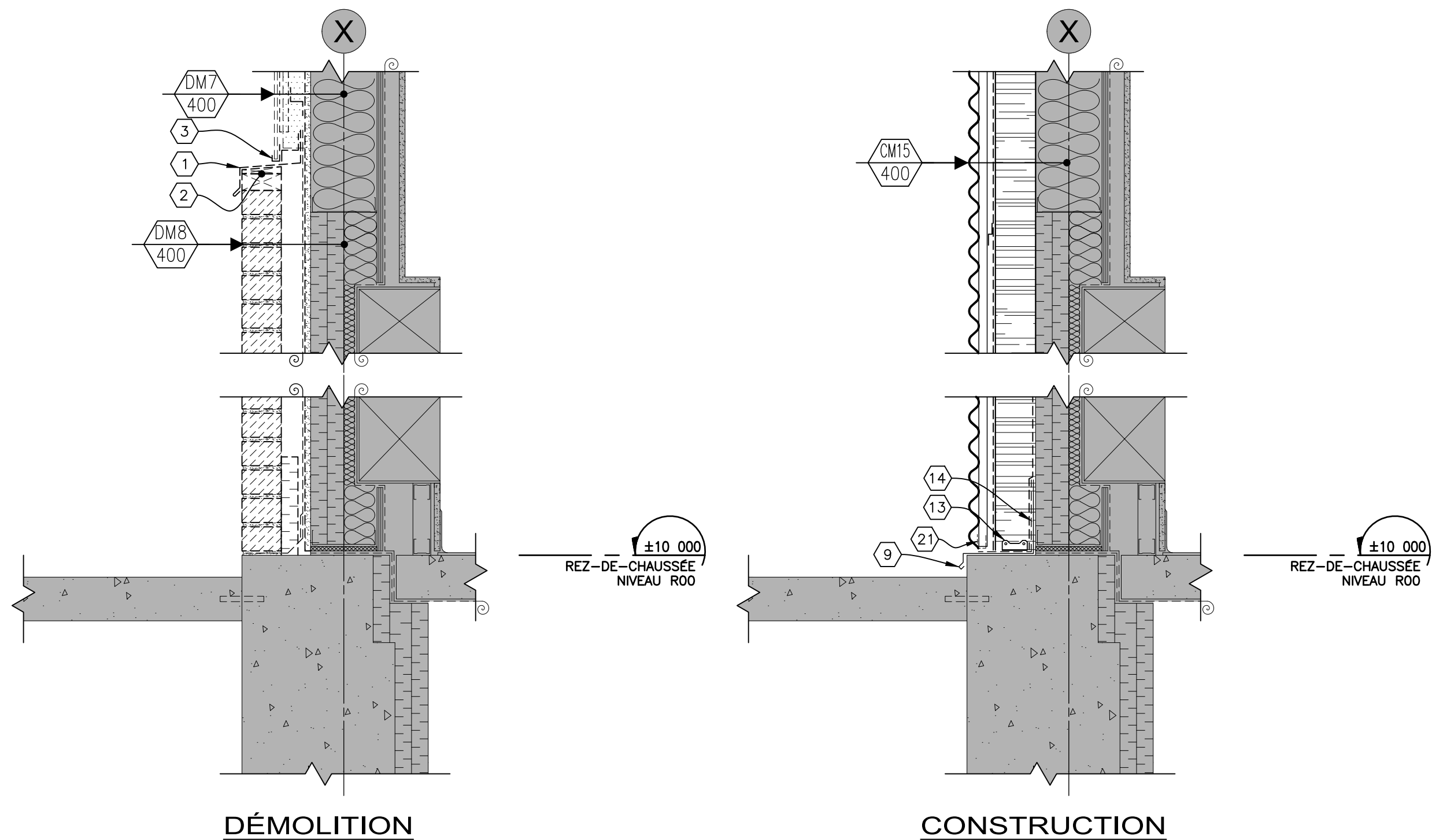
28 DÉTAIL TYPE 407 414 1:10mm (IRM)
