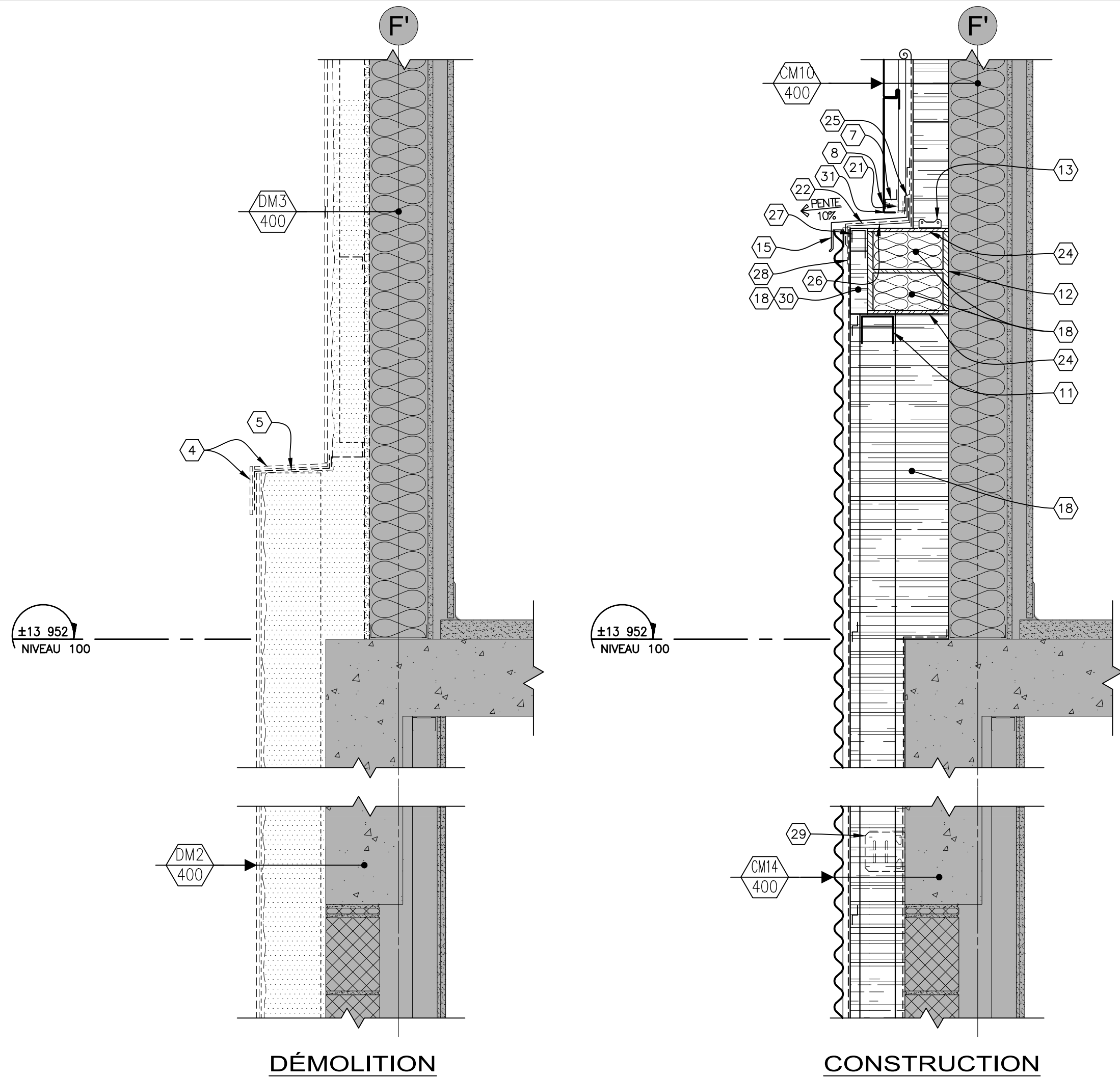
25 DÉTAIL TYPE PARAPET 406,513 414 1:10mm (ADMINISTRATION)
