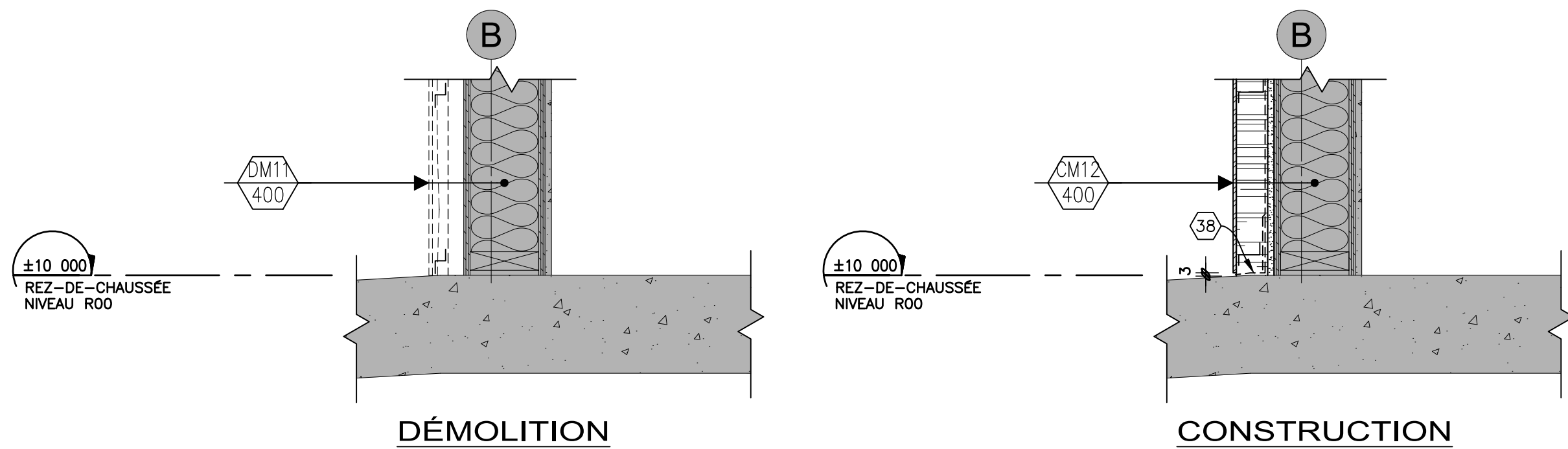
30 DÉTAIL TYPE 407 415 1:10mm (GARAGE AMBULANCE)
